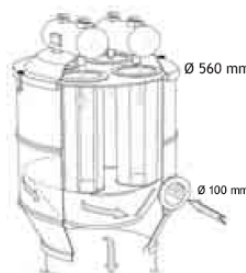
Option cartouche à décolmatage pneumatique
