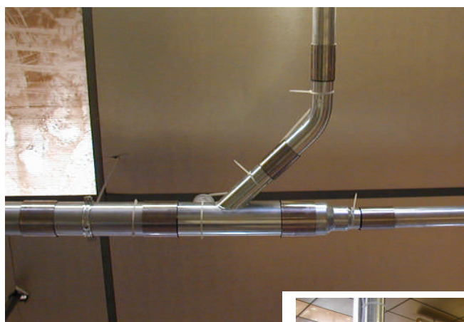
Réseau collecteur en acier
