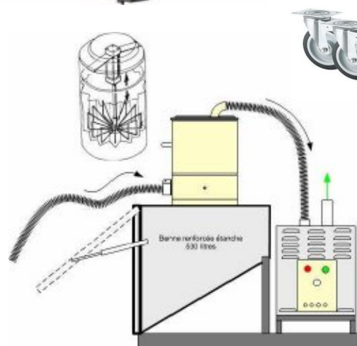
Châssis mobile avec 4 roues
